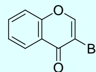
3-Bromochromone
