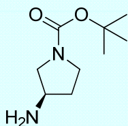
( R )-(+)-1-Boc-3-aminopyrrolidine
