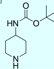
4-( N -Boc-amino)piperidine
