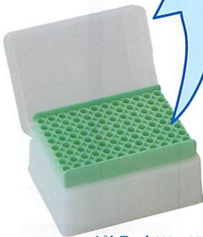
ピタラック(10~250 \mu l) 寸法: 121×95×77(mm)
